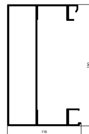
Bočná krokva s prierezom 120×190 mm
