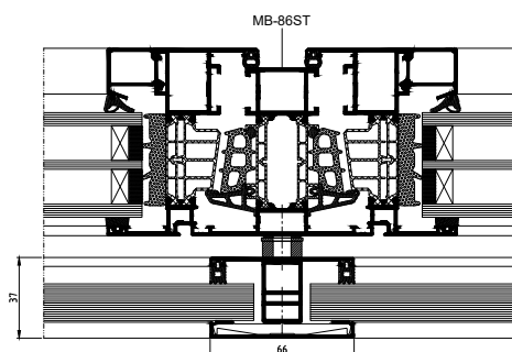
řez středovým sloupkem okna se zábradlím
