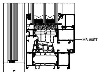
spodní řez okna se zábradlím
