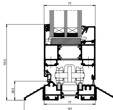
Spodný rez prahu s kombinovaným tesnením
