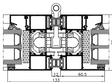
Rez spojením dverných krídiel
